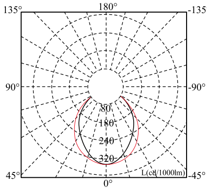
T5 3 x 14W Dimensión de caja: 64x12x63cm Contenido: 2 piezas / caja
