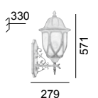
E800W-L farol de muro grande E26 1 x 60W
