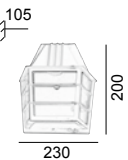
5024A Arbotante para exterior elaborado en aluminio 1x60W E27
