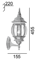
E502 farol de muro A-19 socket Dimensión de caja:81.5x42x34.5cm Contenido: 10 piezas / caja
