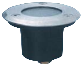
174 •luminario para empotrar en piso •IP 65 •Acero satinado •lámpara recomendada mr11 35W(no incluida) •Tornillería de seguridad •cristal termotemplado •Dimensión de caja:47x23x38cm •Contenido: 20 piezas / caja
