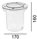
HG171 •luminario para empotrar en piso •IP 68 •Acero satinado y PVC •lámpara recomendada AR111(no incluida) •Tornillería de seguridad •cristal termotemplado •Dimensión de caja:94x20x39cm •Contenido: 10 piezas / caja
