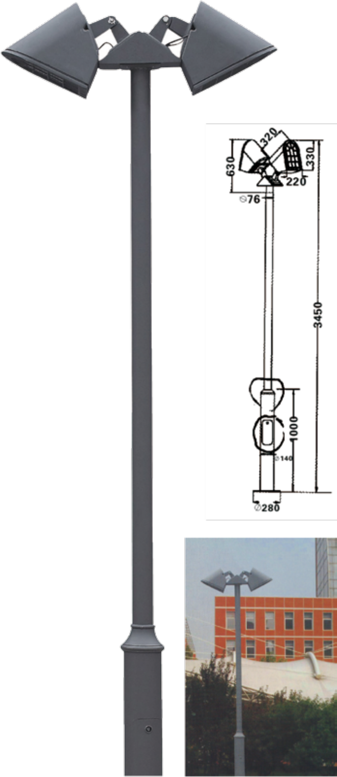
LB-36 Lamp Source: Rx7S Power:70W-150W Material:Aluminium IP55 Dimensión de caja: 300x27x27cm Contenido: 1 piezas / caja Rx7S
