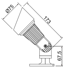
HG-701 ALUMINIO 12V/MR16 50W MAX. Dimensión de caja: 41.5x21.5x43.5cm Contenido: 20 piezas / caja
