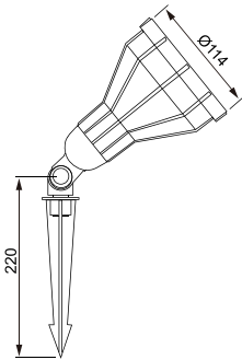
HG-206 FIBRA DE VIDRIO 120V/PAR38 MAX. 100W Dimensión de caja: 76.5x31.5x46.5cm Contenido: 20 piezas / caja
