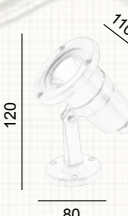
411 lampara elaborada en acero inoxidable Difusor de vidrio templado, class III, IP68, GU5.3, MAX 35W,12V GU5.3 1x35W lumen: 80-90 angulo: 25 IP: 68 material: acero inoxidable
