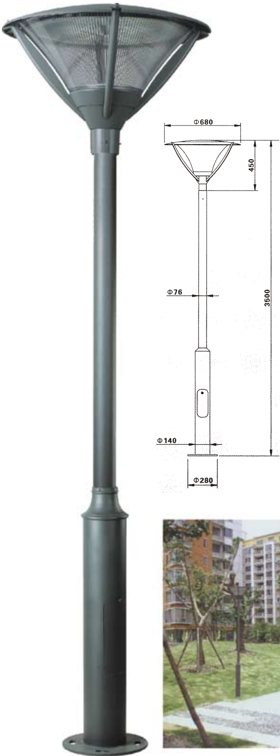
LB-4 Lamp Source: G12 Power:70W-150W Material:Aluminium +PC IP55 Dimensión de caja: 300x27x27cm Contenido: 1 piezas / caja G12
