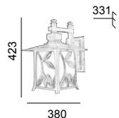
A0219-32 1x 60 Watt arbotante aluminio y cristal A-19
