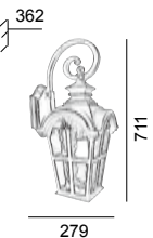
A0244-32 aluminio y cristal socket A-19 127V acabado: bronze antiguo
