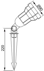
HG-205 FIBRA DE VIDRIO 120V/PAR20 MAX. 100W Dimensión de caja: 51.5x21.5x43.5cm Contenido: 20 piezas / caja
