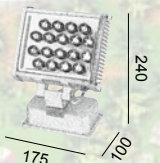
TGD LED PARA EXTERIOR 1X18W angulo: 30 IP: 65 disponible en color de Led: Blanco Calido y Rgb material: Aluminio,Vidrio
